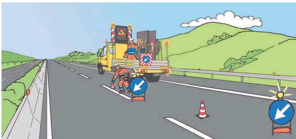
Figura 33 – Chiusura della corsia di marcia: inizio della posa dei coni
